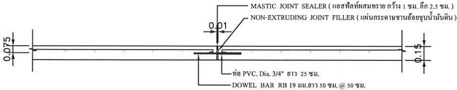
EXPANSION JOINT (ใส่ทุกความยาว 50.00 ม.)
