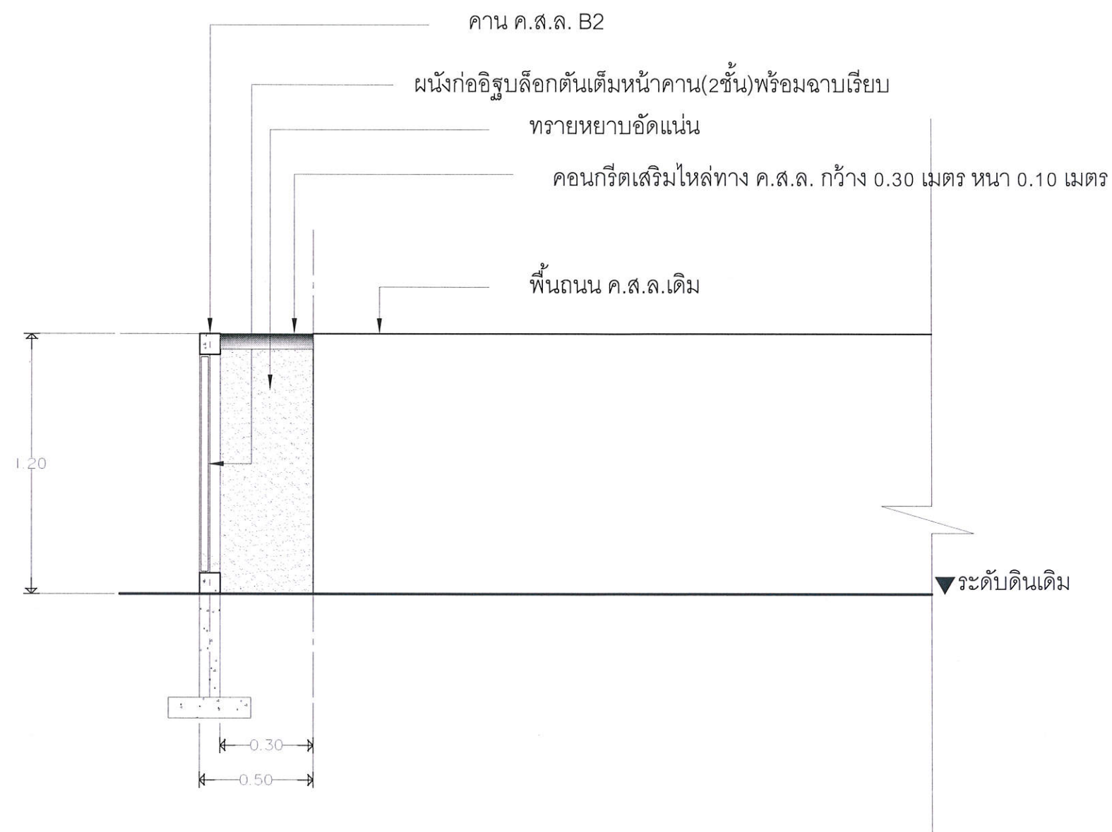
รูปด้านผนังกันดิน ยาว 5.00 เมตร(แบบขยายที่ 2)
