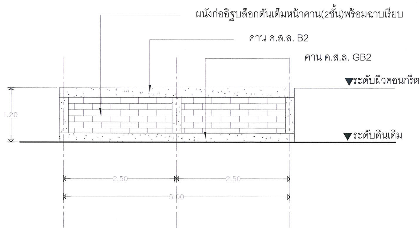
รูปด้านผนังกันดิน ยาว 5.00 เมตร(แบบขยายที่ 2)
