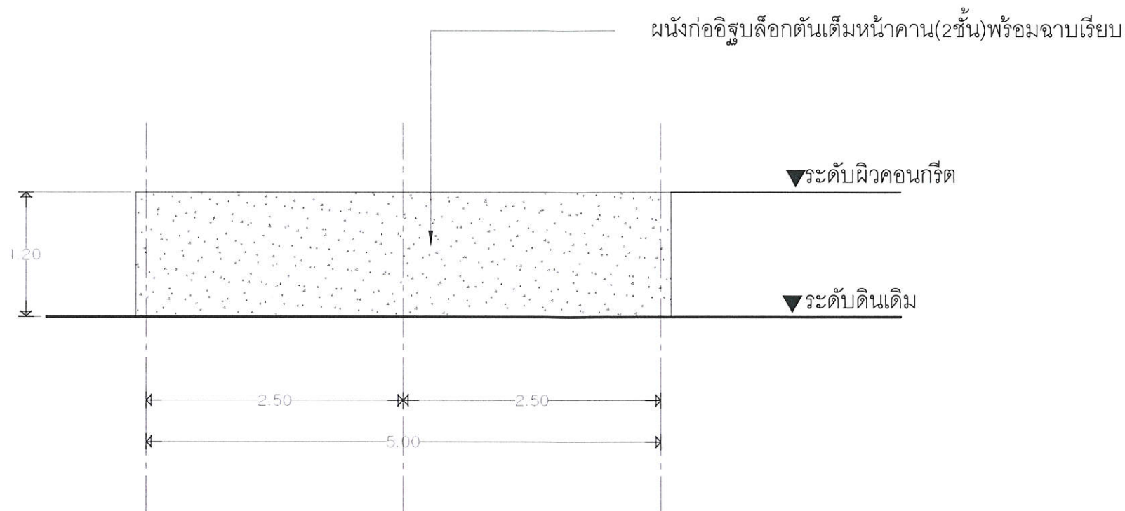
รูปด้านผนังกันดิน ยาว 5.00 เมตร(แบบขยายที่ 2)
